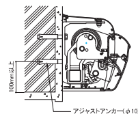
▼ALC造壁面納まり
