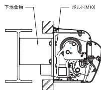
▼ALC造壁面納まり
