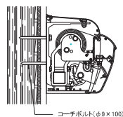
▼木造壁面納まり
