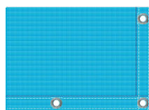
周囲折り返し二本針 ミシン縫製ハトメ打ち
